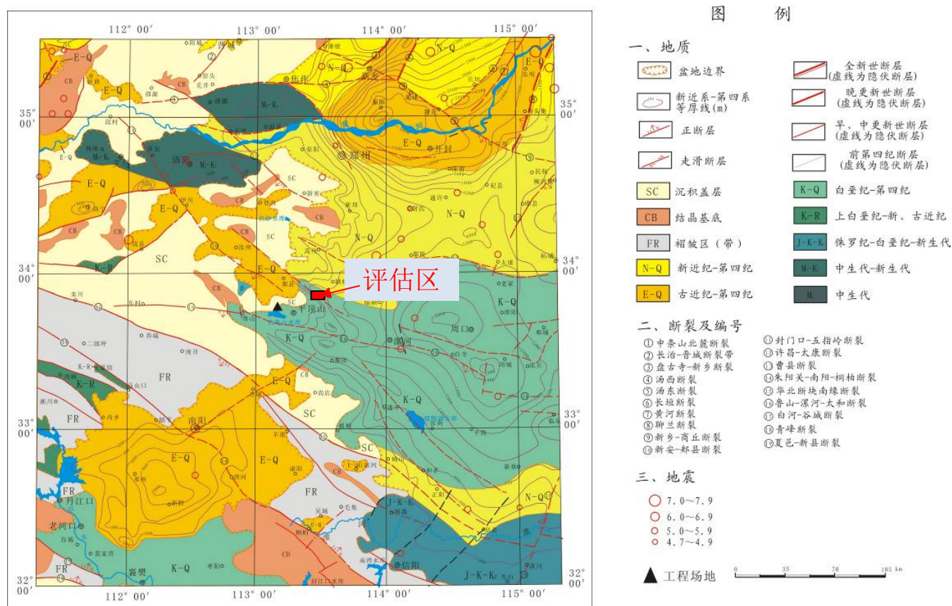
图 2-4 区域地震构造图
